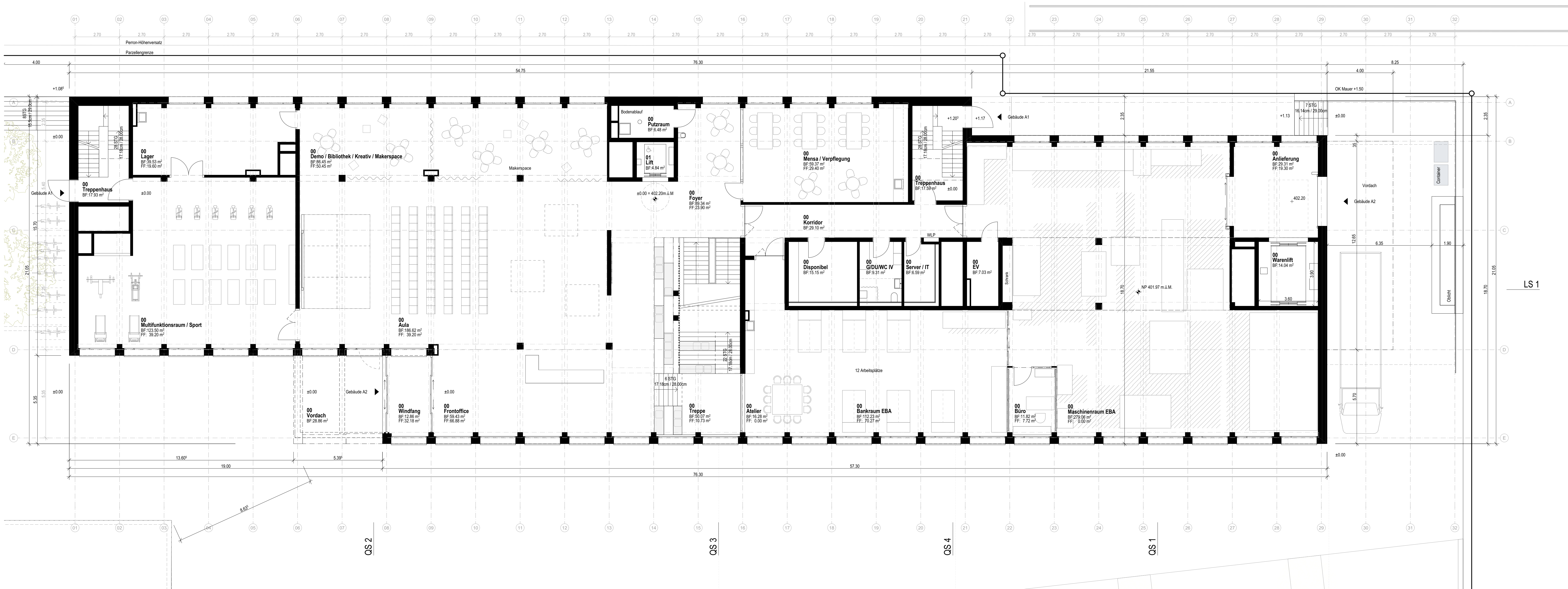
Erdgeschoss
