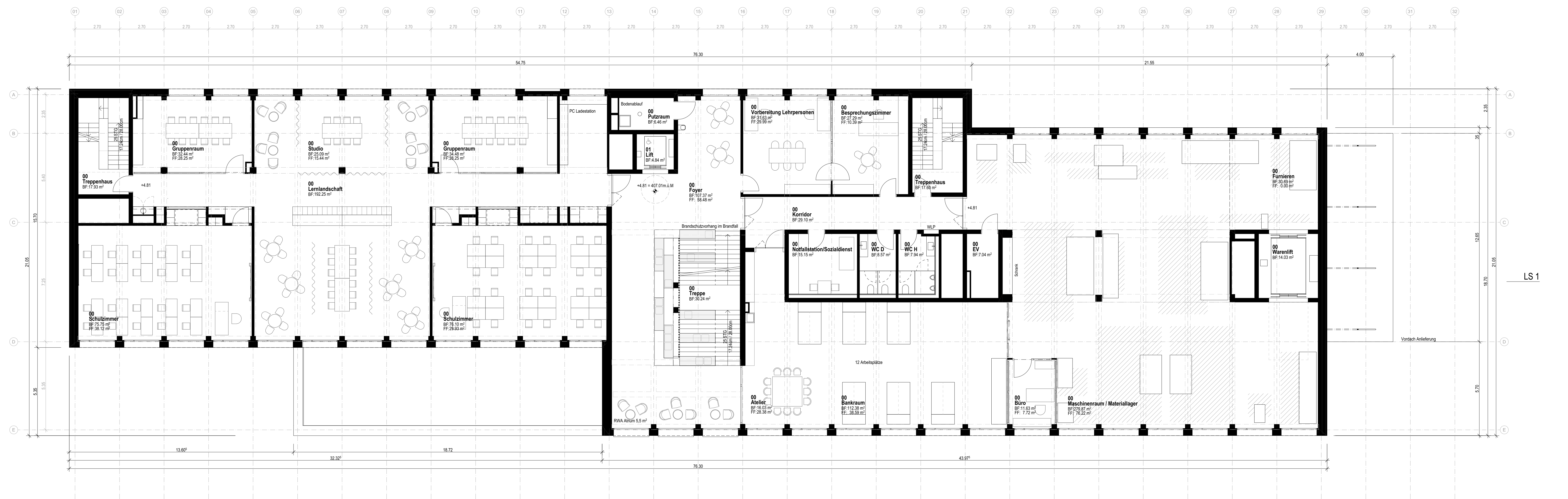
1. Obergeschoss
